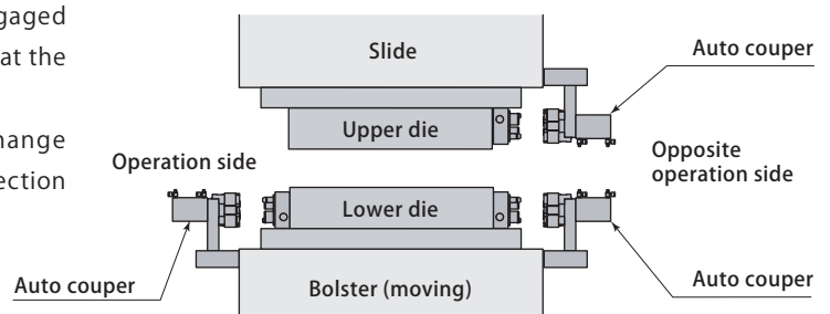
1200ton hot press
