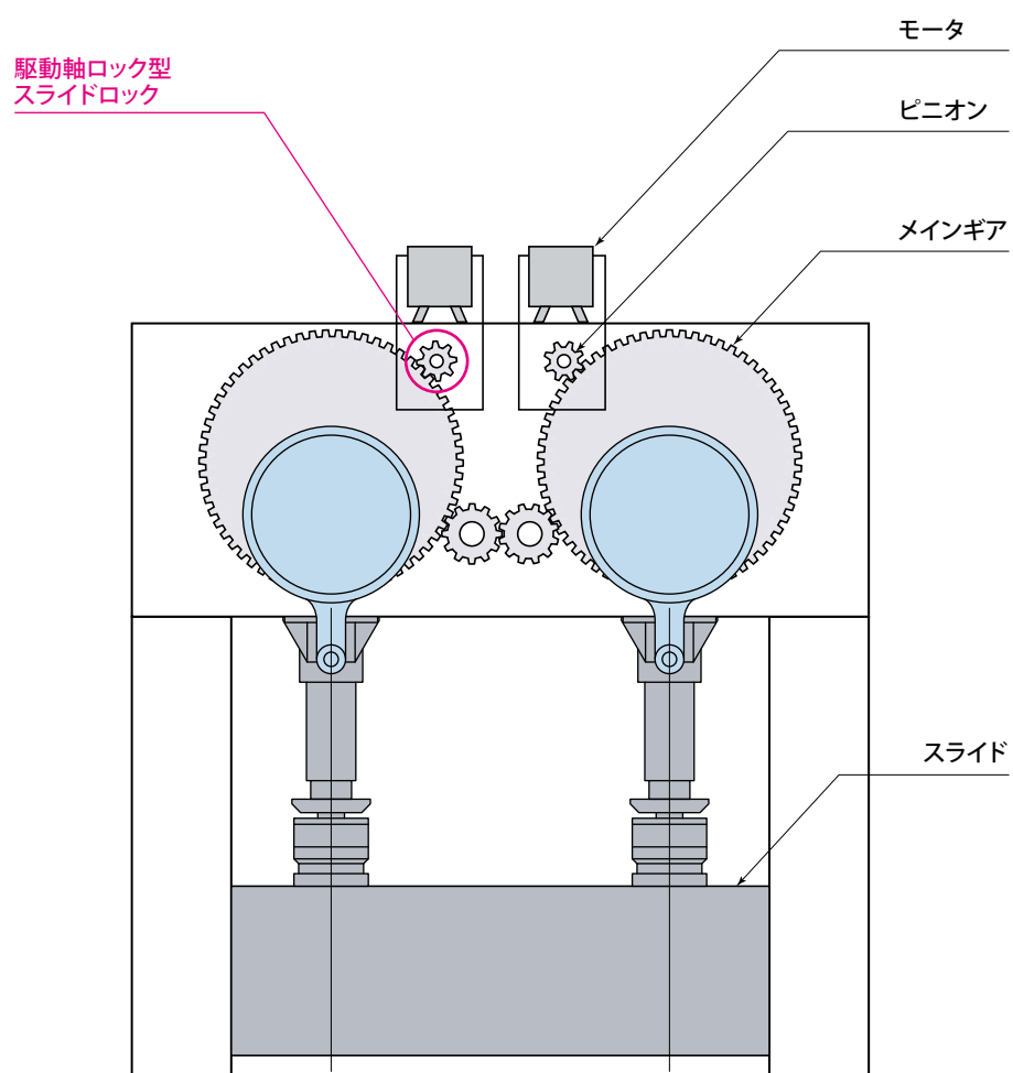
プレス機械
