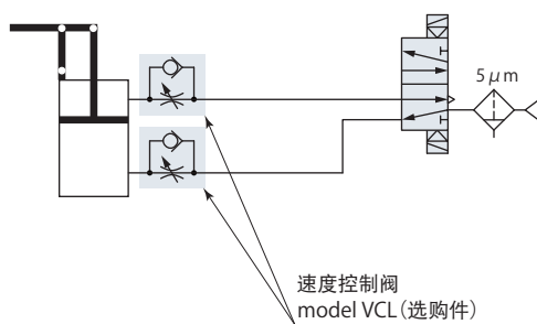
气压回路图
