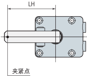
标准夹紧臂
