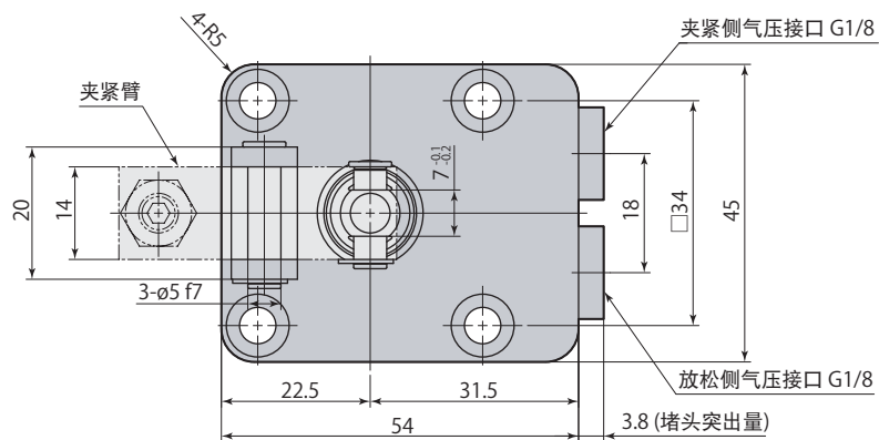
外形尺寸图
