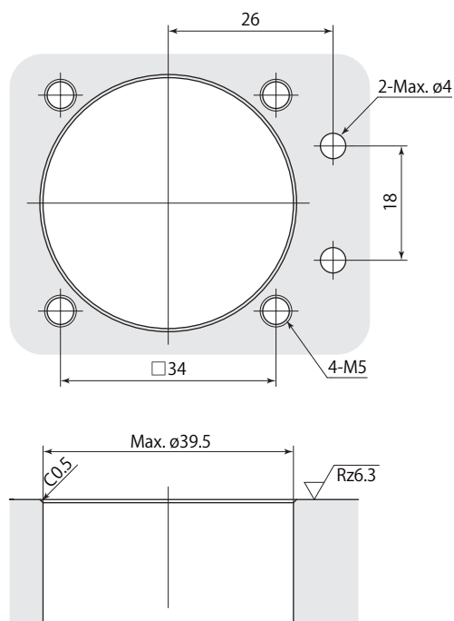
安装孔加工图
