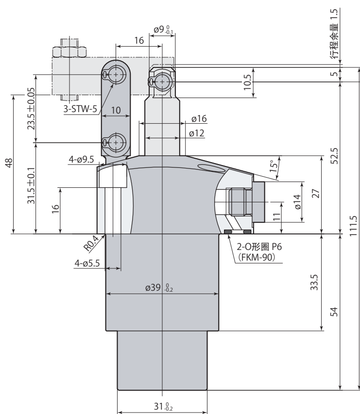
夹紧
