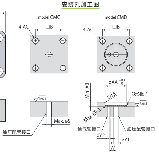
※: 与拉式夹紧器本体一起包装的O形圈, 请在使用法兰盘时安装。
